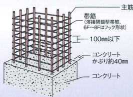
●柱構造イメージイラスト
